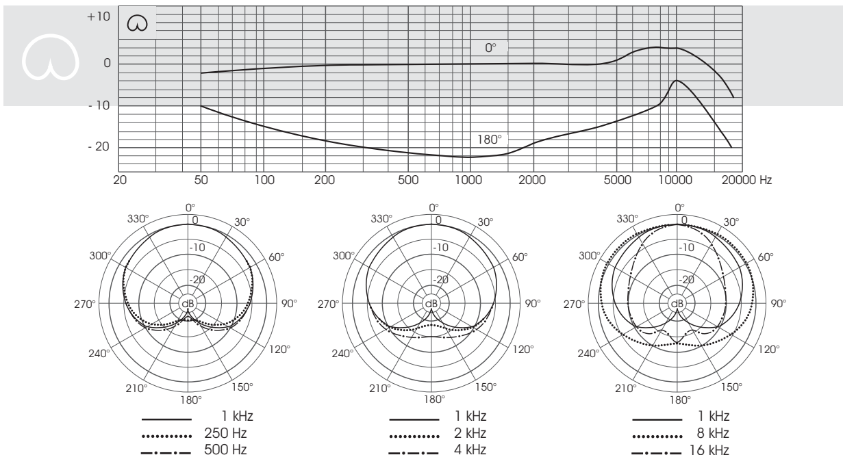
dB Frequenzgänge TM 190
